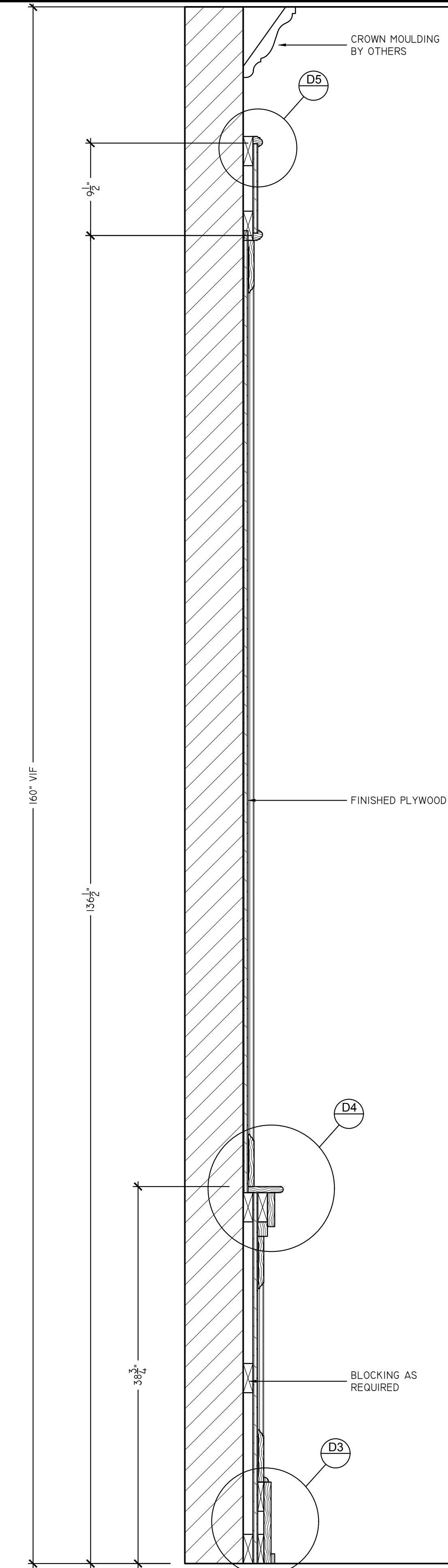
SI TYPICAL COLUMN - SECTION SCALE: 1-1/2\"/>
