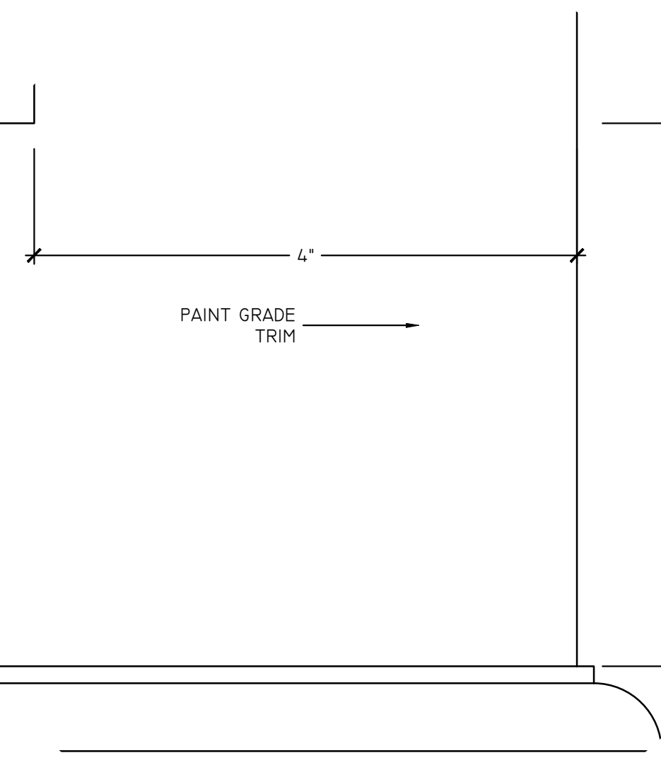
D1 TYPICAL COLUMN - DETAIL SCALE: 1'-0\"/>
